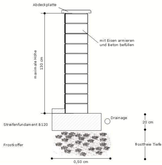
Aufbau einer Böschung – Schnitt mit Streifenfundament
